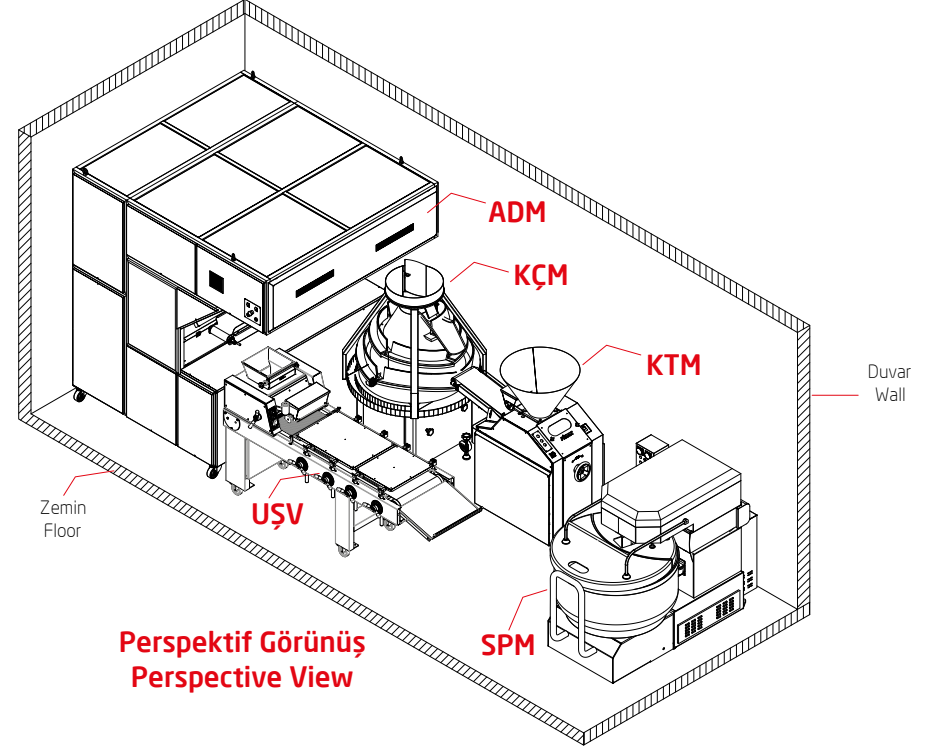
Perspektif Görünüş Perspective View
