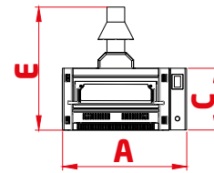
Ön Görünüş Front View
