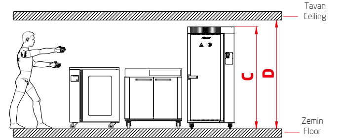
Sol Yan Görünüş Left Side View
