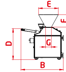
Sağ Yan Görünüş Right Side View
