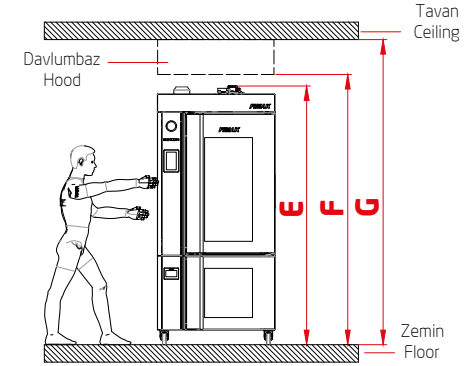
Montaj Boşlukları Mounting Holes
