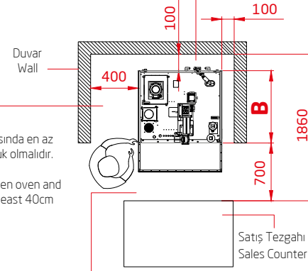
Montaj Boşlukları Mounting Holes
