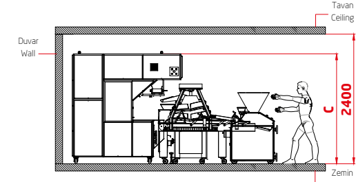
Montaj Boşlukları Mounting Holes
